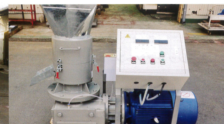
TM-PM350S-22型 (ペレットマシン) 駆動29馬力(3相200V-22 kw) 能力250K~350K/H
