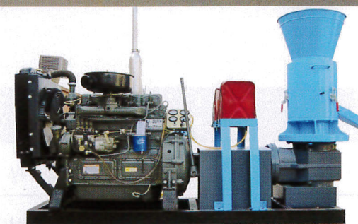
TM-PM350E-22型( 硬化質ペレットマシン) 軽油式4気筒ディーゼルエンジン付き能力250K~350K/H
